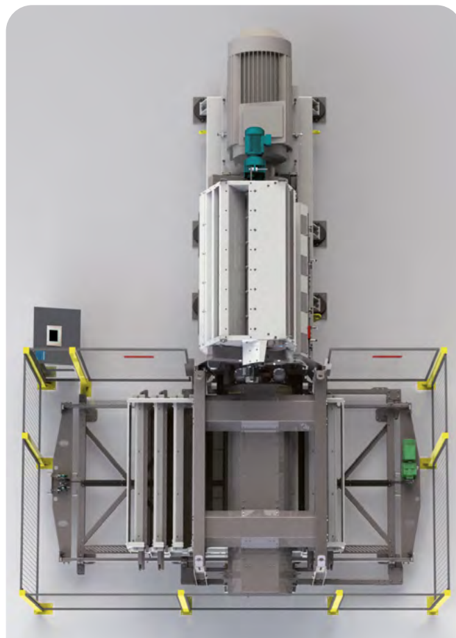
Translation du chariot (version 4 grilles)
